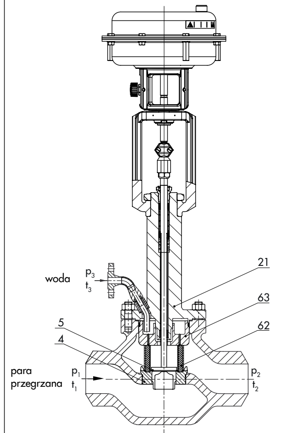
Rys. 4 - Zawór redukcyjno-schładzający do pary, typu 3281-7, z elementem izolującym, końcówkami do spawania i z siłownikiem typu 3277
