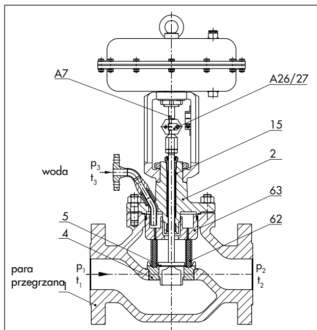
Rys. 3 - Zawór redukcyjno-schładzający do pary, typu 3281-1, z przyłączem kotłowym i siłownikiem typu 3271
