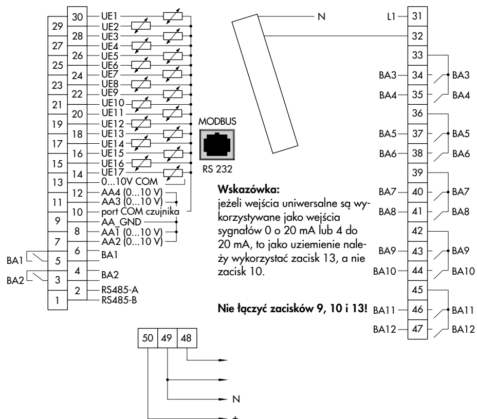
Rys. 2 · Przyporządkowanie zacisków sterownika swobodnie programowalnego TROVIS 5571
