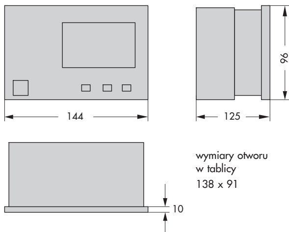
Rys. 7 · TROVIS 5479
