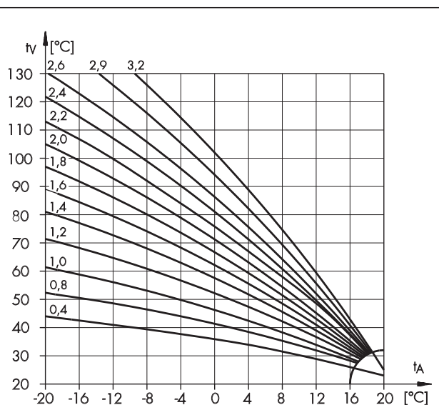
Rys. 4 · Krzywe grzania
