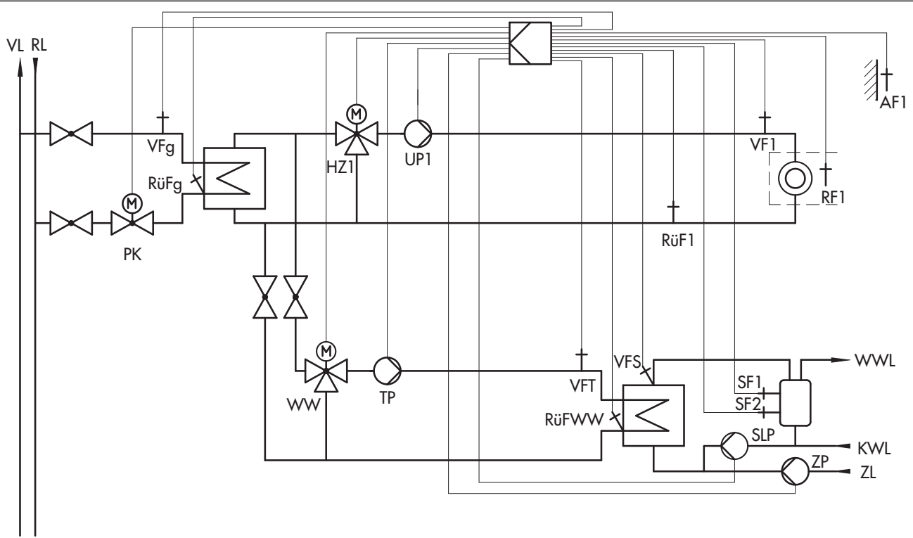
Rys. 9 · Instalacja nr 4
