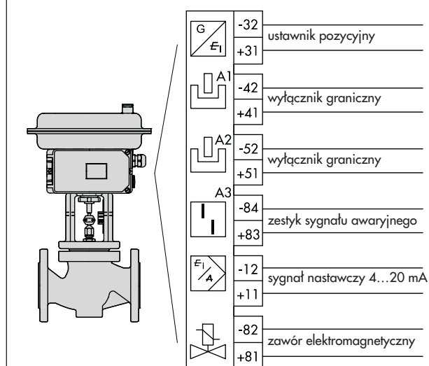
Rys. 3 · Opcjonalne wyposażenie ustawnika pozycyjnego
