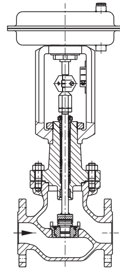
Rys. 3 · Zawór typu 3251-1 z ceramicznymi elementami nastawczymi
