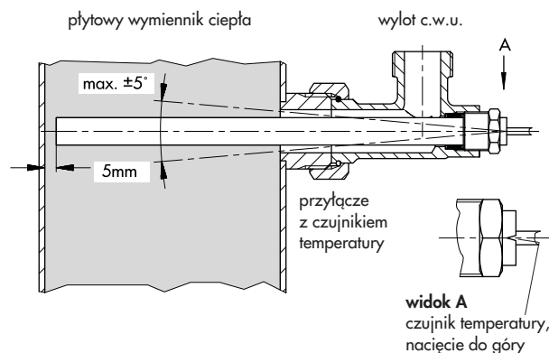
Rys. 3 · Montaż czujnika
