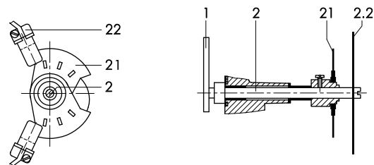
Bild 4 · Ausführung mit zwei induktiven Grenzkontakten
