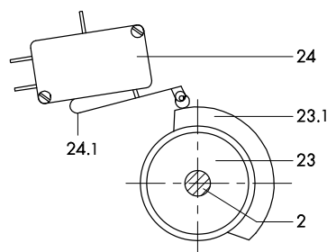
Bild 6 · Wirkbild der Ausführung mit einem elektrischen Grenzkontakt
