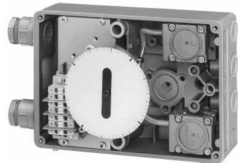
Bild 3 · Grenzsignalgeber mit Magnetventil Typ 3775-11 (ohne Gehäusedeckel)
